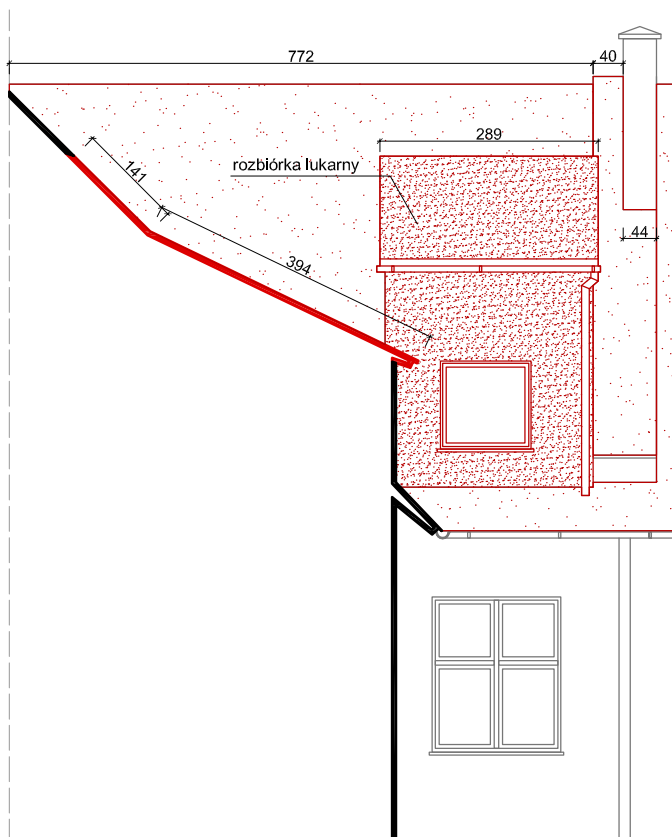
WIDOK C-C
